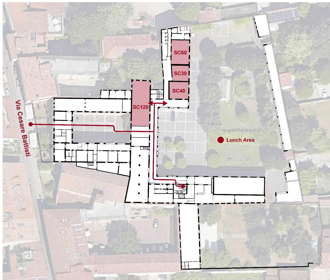
Pianta del piano Terra
